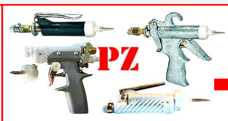
PZ™-TÜÜPI KÄSIPÜSTOLID
